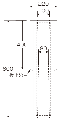
Kタイプ柱
